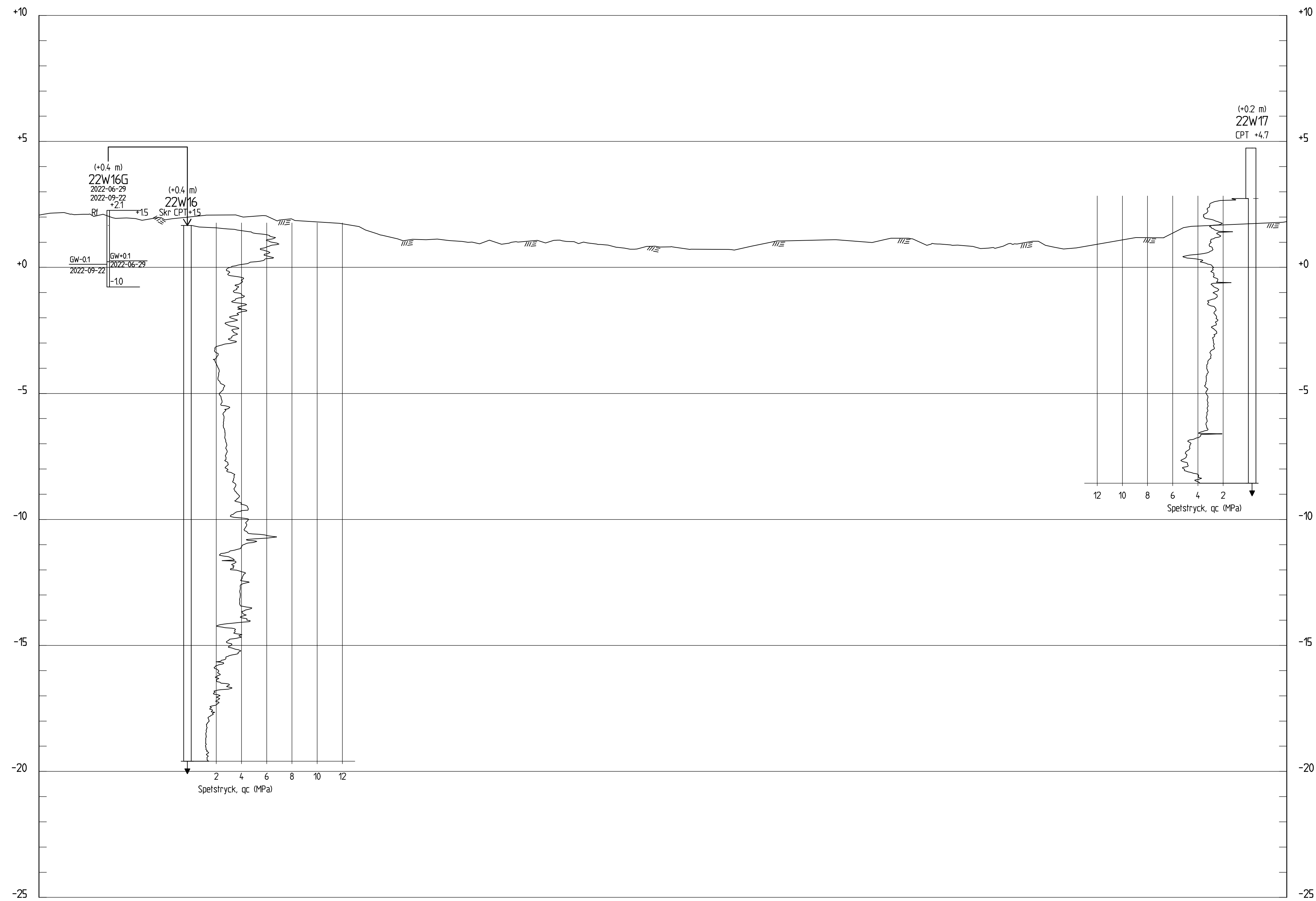
SEKTION J-J H 1: 100 L 1: 200
